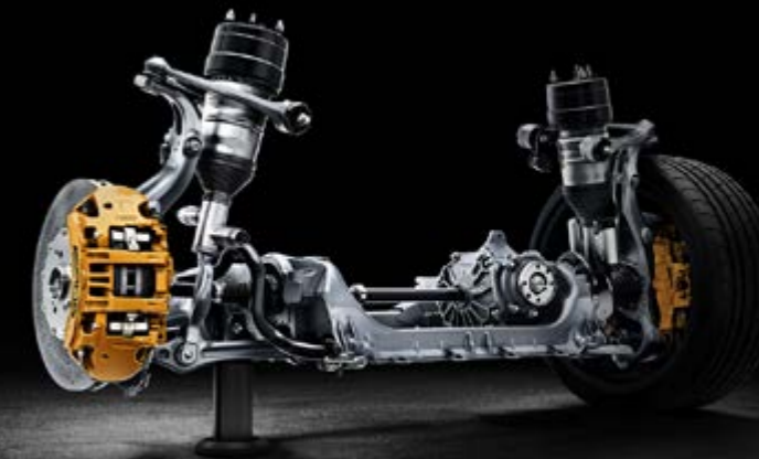
489 – Fahrwerk AMG RIDE CONTROL+
