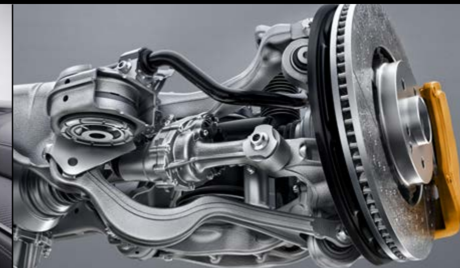
201 – Hinterachslenkung
