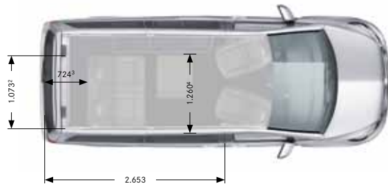
Bank in Sitzposition
