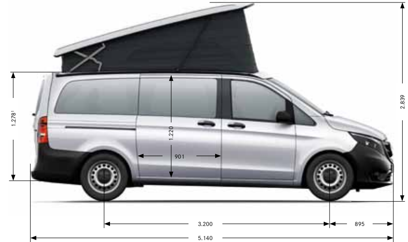
Seitenansicht mit geöffnetem Aufstelldach
